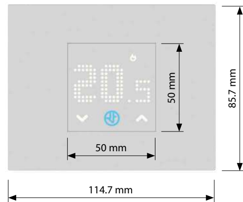
Montage auf 3-Modul-Box
