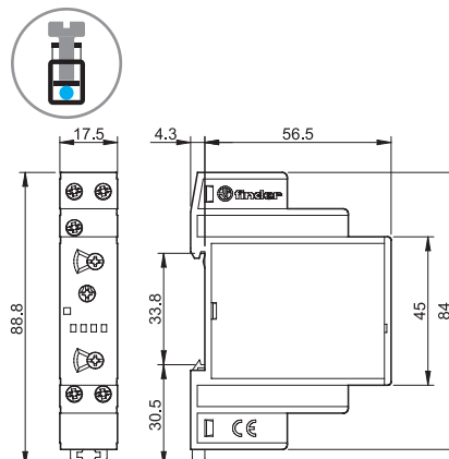
Typ 80.71 Zaciski śrubowe
