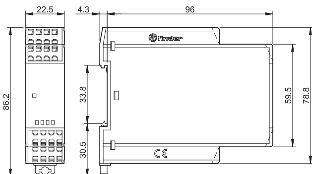
Tipo 75.32 Morsetti a bussola
