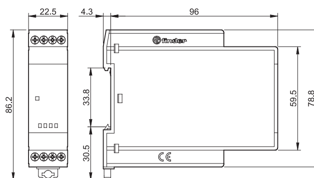
Tipo 75.36 Morsetti a bussola
