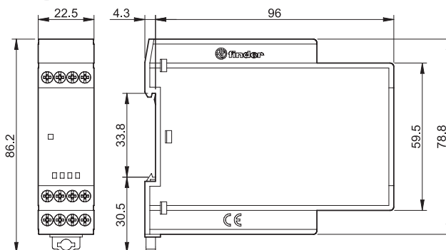
Tipo 75.63 Morsetti a bussola
