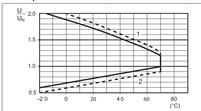
R 7S - Campo di funzionamento bobina DC in funzione della temperatura ambiente - 7S.12/32 / 7S.23 / 7S.14/34 / 7S.16/36
