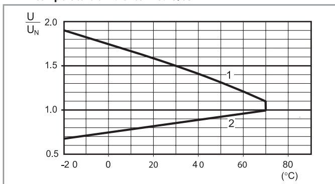
R 7S - Campo di funzionamento bobina DC in funzione della temperatura ambiente - 7S.43/63
