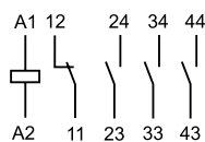
7S.14...4310
