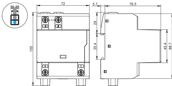
類型 7P. 13. 9. 000. x006 螺絲端子
