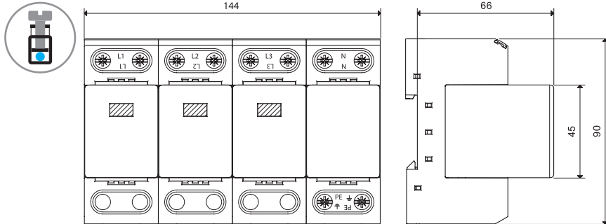
類型 7P. 04 螺絲端子
