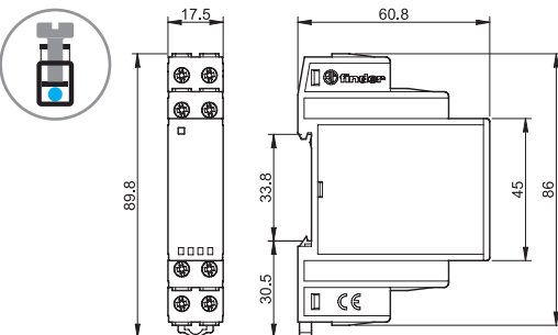
類型 7P. 37. 8. 275. 1003 螺絲端子
