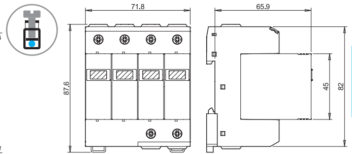
類型 7P. 25 / 7P. 45 螺絲端子
