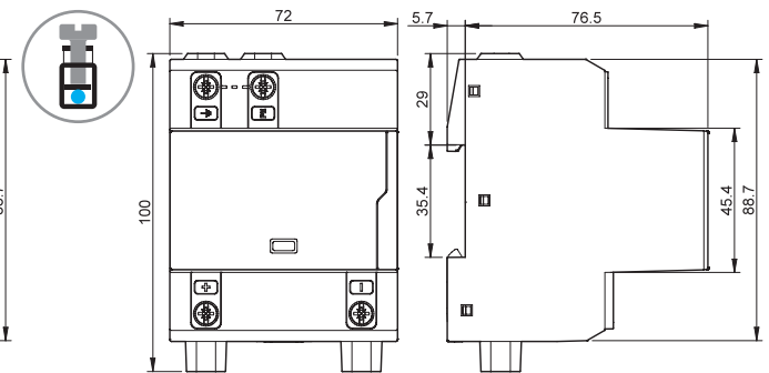
類型 7P. 13. 9. 500. x006 螺絲端子
