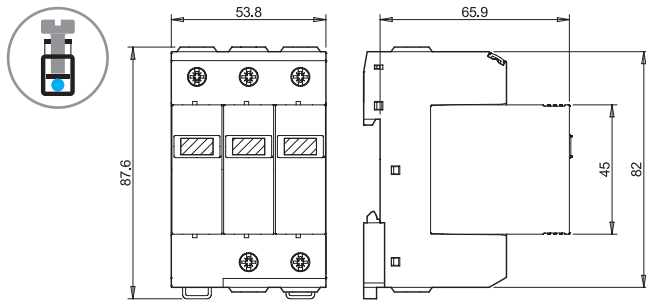
類型 7P. 23. 8 / 7P. 43 螺絲端子
