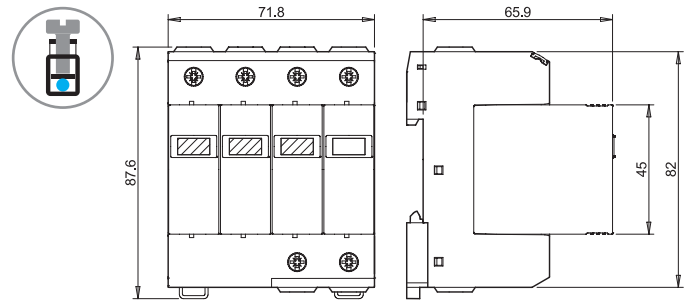
類型 7P. 24 / 7P. 44 螺絲端子
