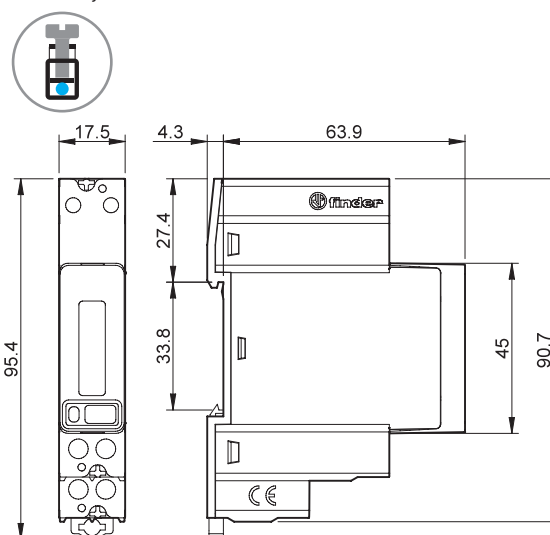
Tipo 7M.24.8.230.0110 Bornes de jaula
