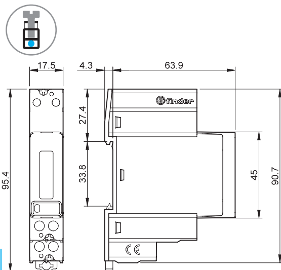
Tipo 7M.24.8.230.0001 Bornes de jaula
