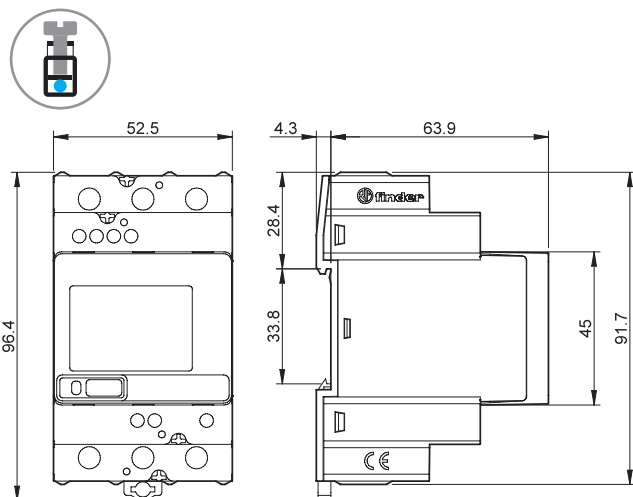
Tipo 7M.38.8.400.0312 Bornes de jaula
