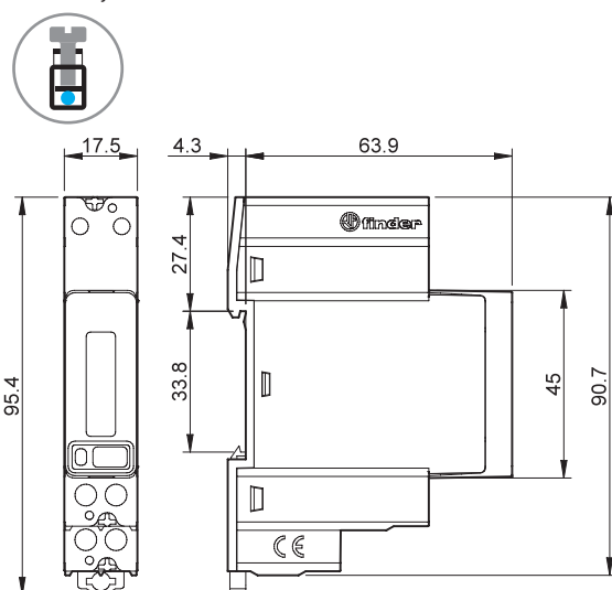
Tipo 7M.24.8.230.0010 Bornes de jaula
