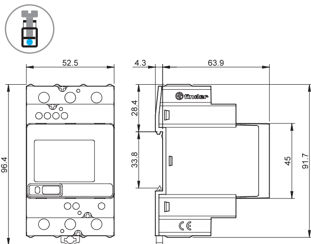
Tipo 7M.38.8.400.0112 Bornes de jaula
