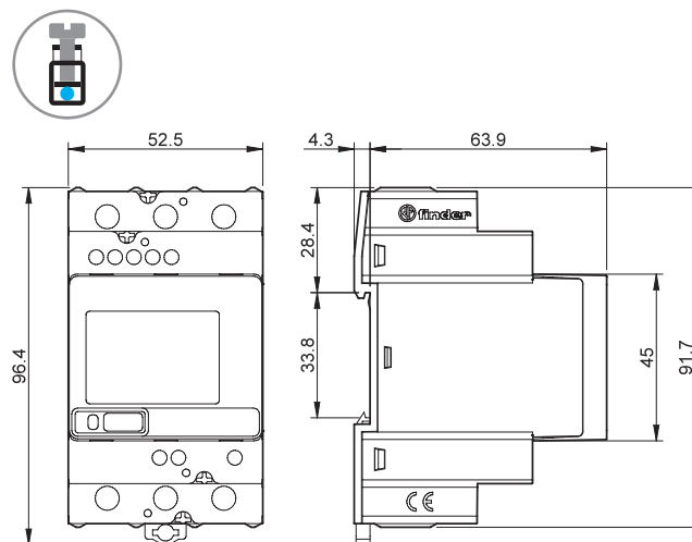
Tipo 7M.38.8.400.0212 Bornes de jaula
