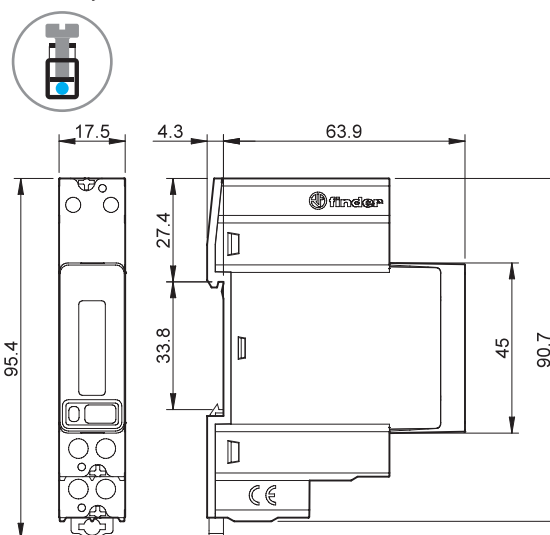
Tipo 7M.24.8.230.0310 Bornes de jaula
