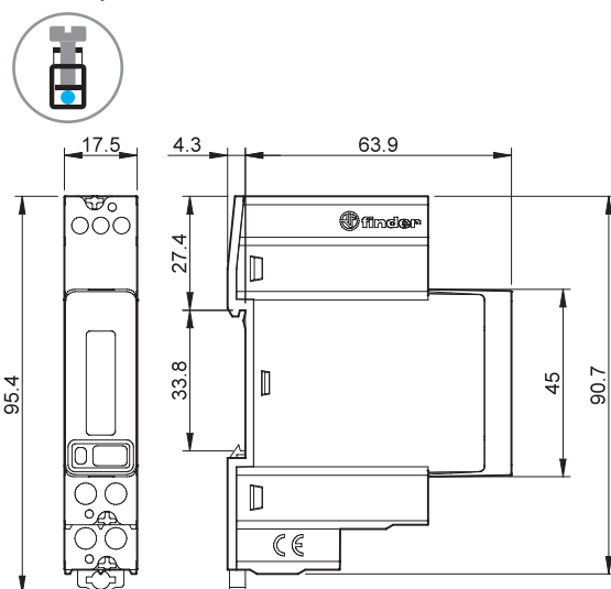
Tipo 7M.24.8.230.0210 Bornes de jaula
