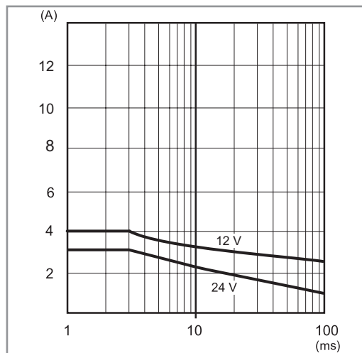
P78-3 Pic de courant en fonction du temps (78.36) 12 V
