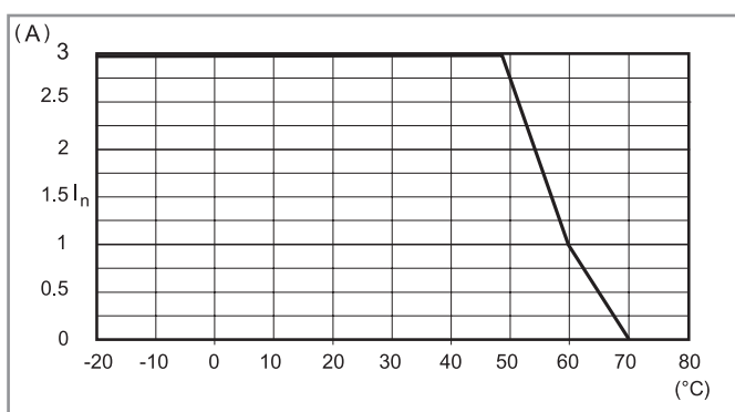
L78-3 Courant de sortie en fonction de la température ambiante (78.36) 12 V
