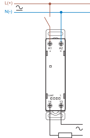
Connexion monophasée (77.11/77.21)
