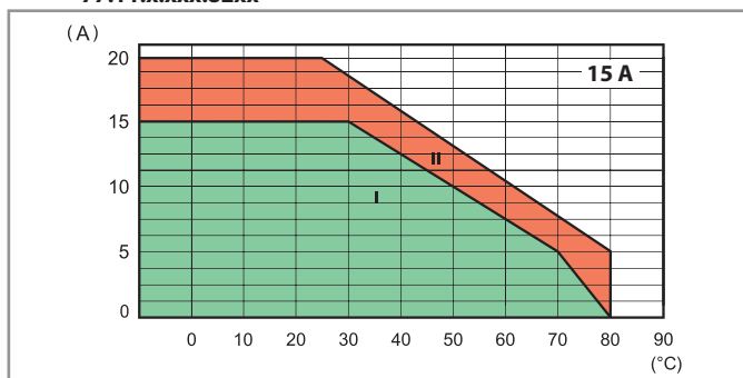
L77-5 Courant RMS en fonction de la température ambiante 77.11.x.xxx.82xx
