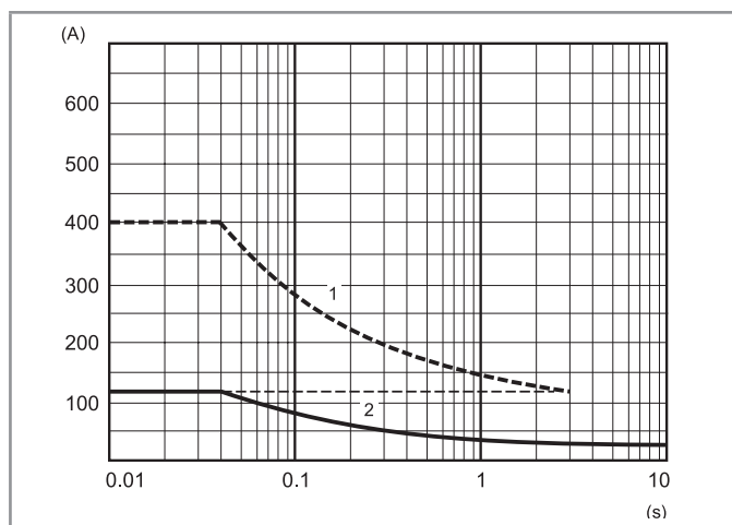
L77-10 Pic de courant (AC) en fonction du temps 77.21.x.xxx.825x
