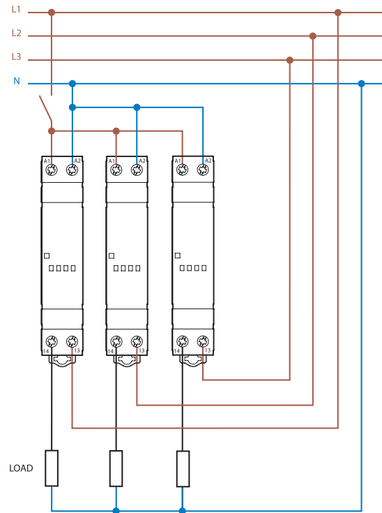
Exemple de connexion triphasée (avec 3 x 77.01)
