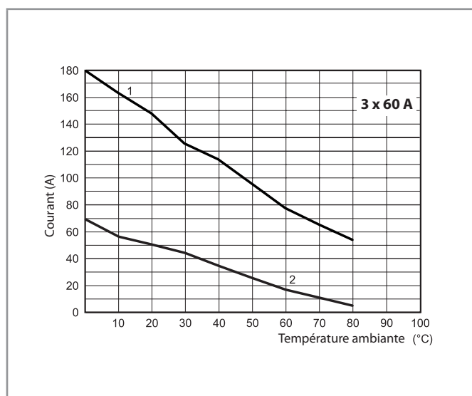
L77-23 Courant RMS en fonction de la température ambiante 77.D3.x.xxx.8671
