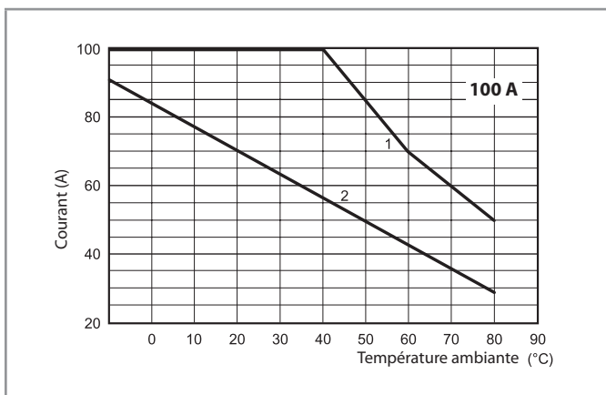
L77-17 Courant RMS en fonction de la température ambiante 77.G1.x.xxx.8x50
