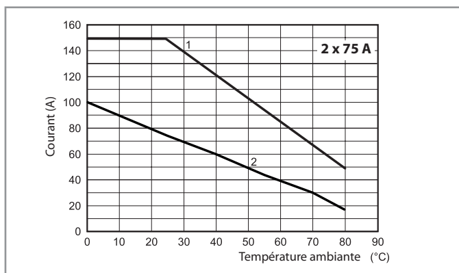
L77-20 Courant RMS en fonction de la température ambiante 77.E2.9.024.8671
