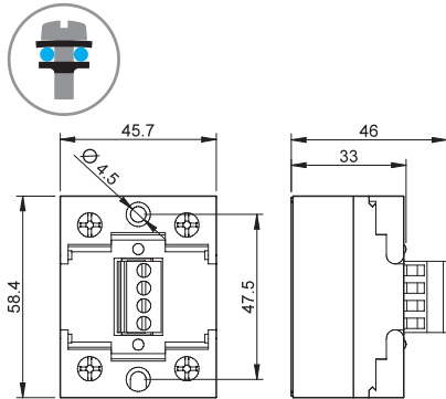
Type 77.x2 Bornes à vis
