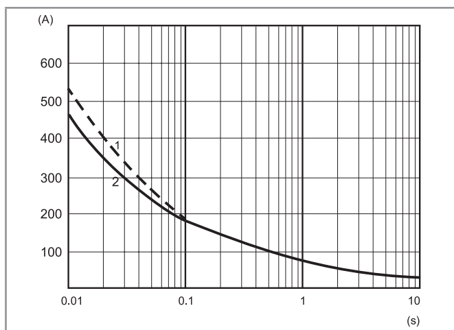
L77-11 Pic de courant (AC) en fonction du temps 77.31.x.xxx.80xx
