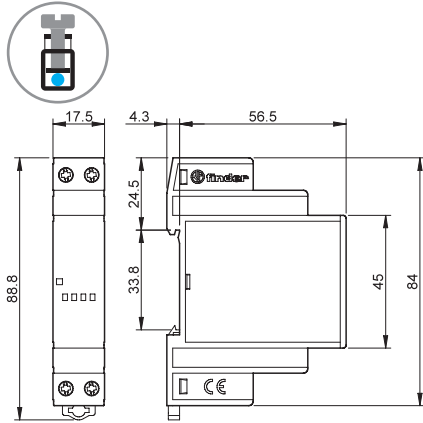
Type 77.01 Bornes à cage
