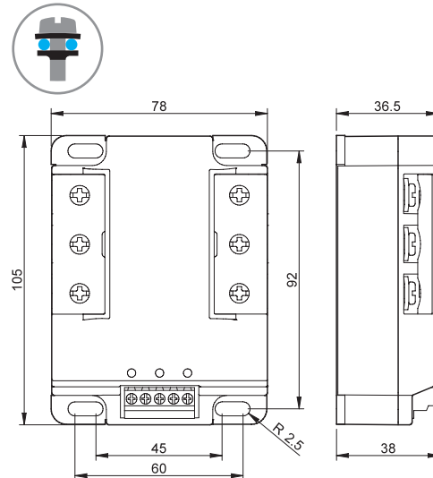
Type 77.x3 Bornes à vis
