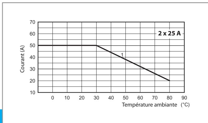
L77-18 Courant RMS en fonction de la température ambiante 77.A2.9.024.8671
