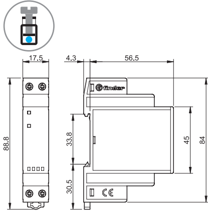
Type 77.x2 Bornes à vis
