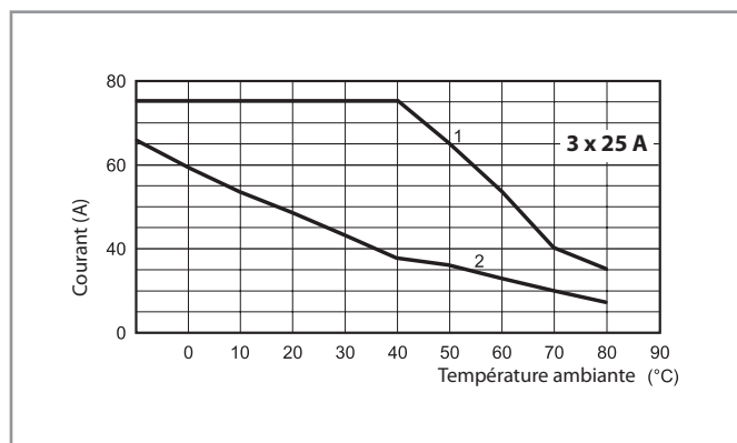
L77-21 Courant RMS en fonction de la température ambiante 77.A3.x.xxx.8671
