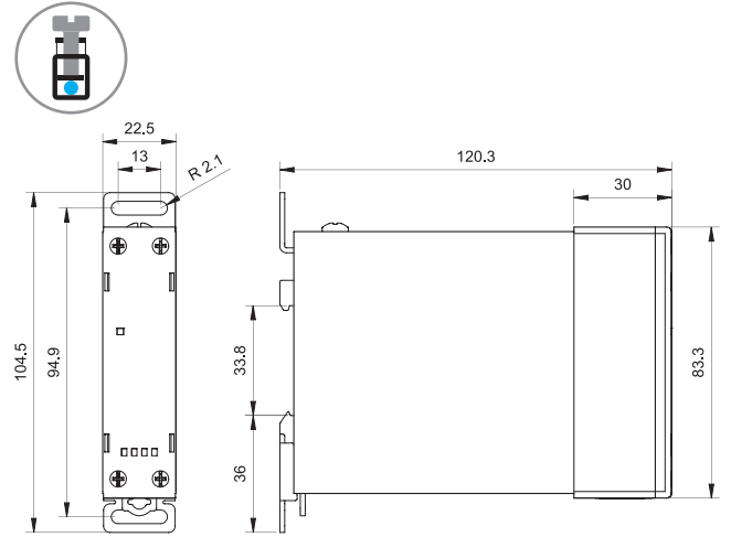
Type 77.x1 Bornes à vis
