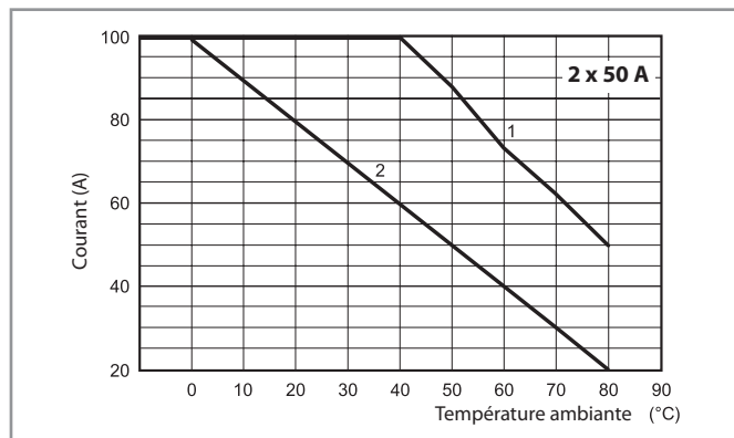
L77-19 Courant RMS en fonction de la température ambiante 77.C2.9.024.8671
