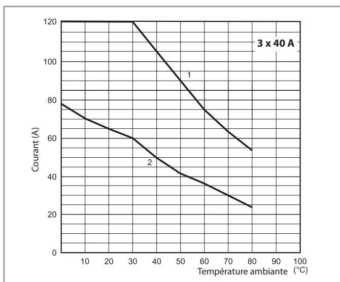
L77-22 Courant RMS en fonction de la température ambiante 77.B3.x.xxx.8671
