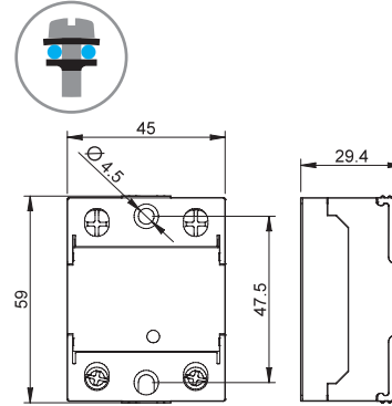
Type 77.x1 Bornes à vis
