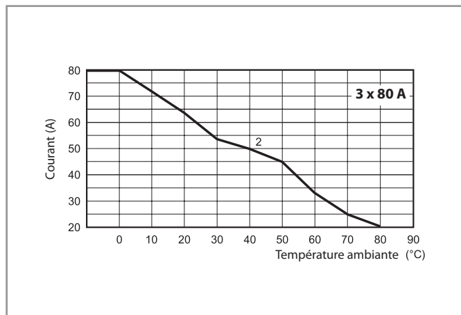
2 - Installation avec dissipateur thermique 077.08 (0.8 K/W)
