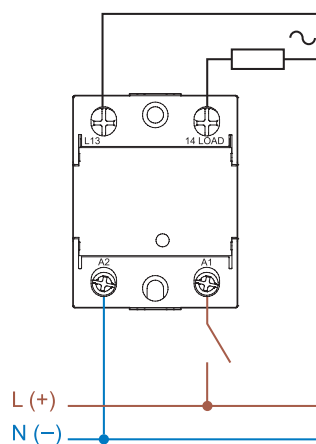
Connexion monophasée (77.x1)
