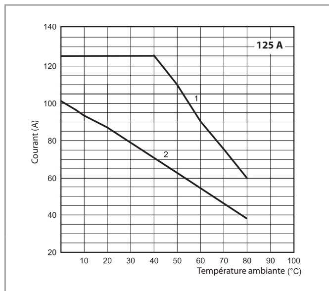
L77-18 Courant RMS en fonction de la température ambiante 77.H1.x.xxx.8x50
