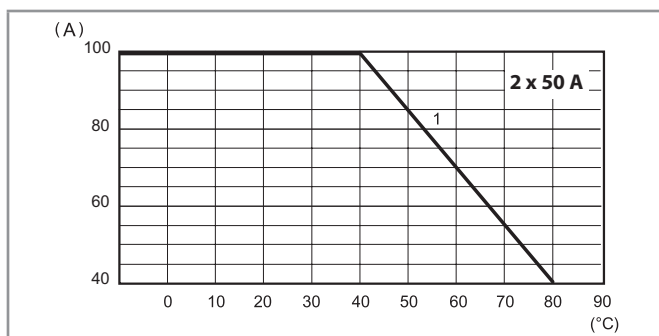
L77-20 Courant RMS en fonction de la température ambiante 77.C2.9.024.8671
