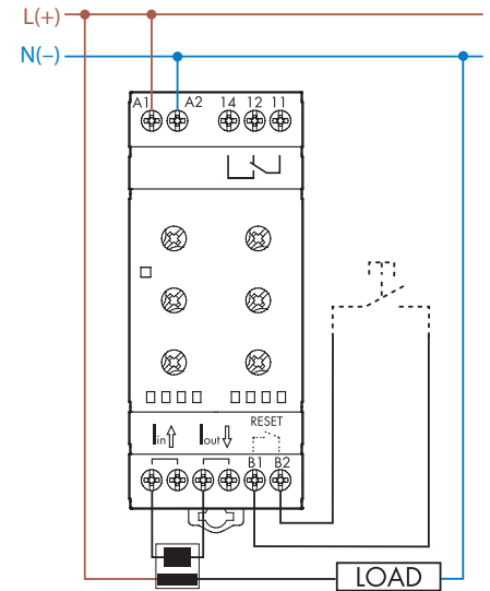
Tipul 70.51 cu transformator de curent - TA
