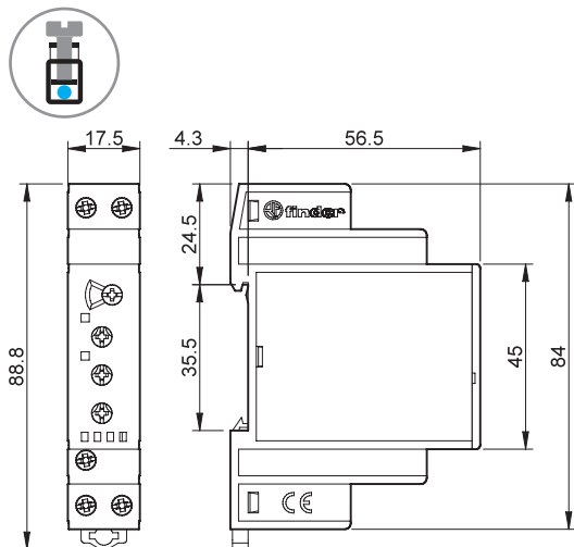
Tipul 70.41 Terminale cu șurub
