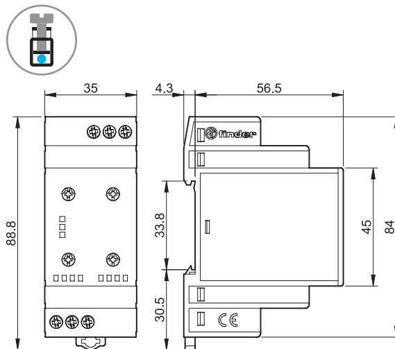
Tipul 70.42 Terminale cu șurub
