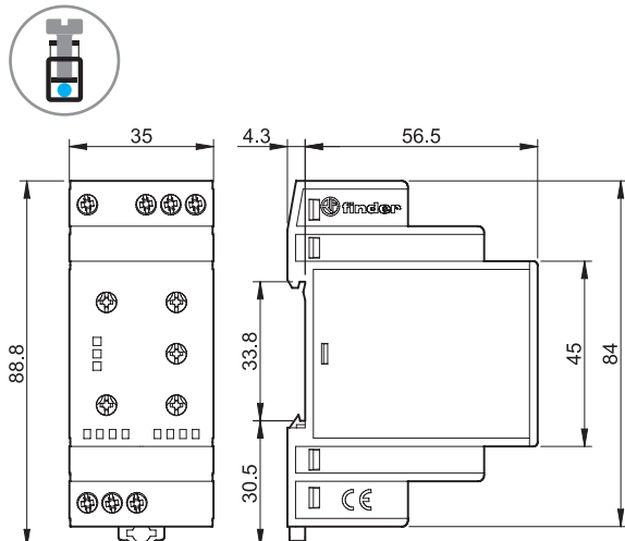
Tipul 70.41 Terminale cu șurub
