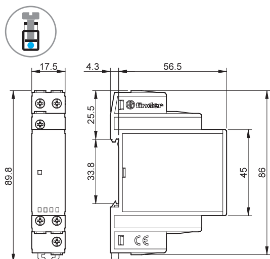
Tipo 70.61 Morsetti a bussola
