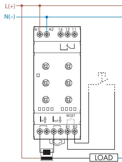
Tipo 70.51 con collegamento TA
