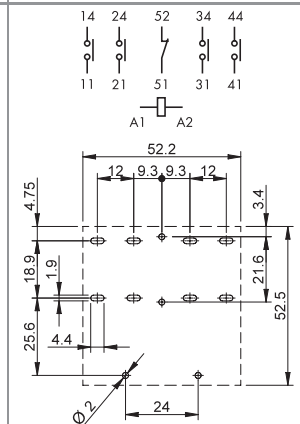
Aanzicht op de aansluitingen*
