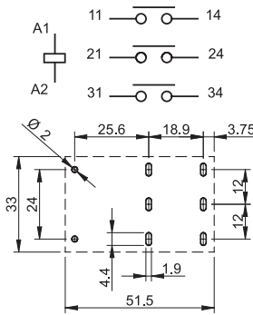
Vue côté cuivre
