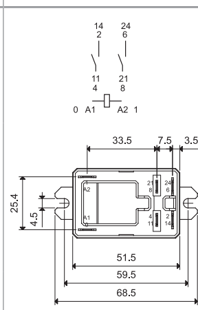
Rysunek otworów montażowych
