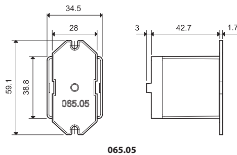
Adaptateur avec patte sur le dessus, pour types 65.31.xxx.xxx9
