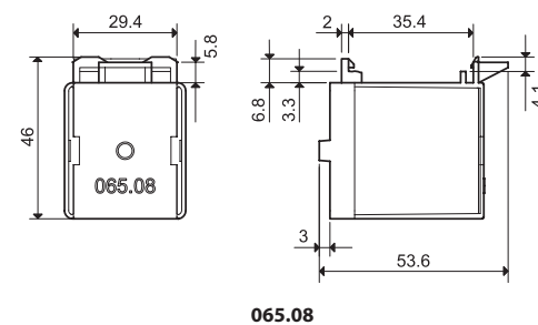
Adaptateur rail 35 mm (EN 60715) à l'arrière pour types 65.31.xxx.xxx9
