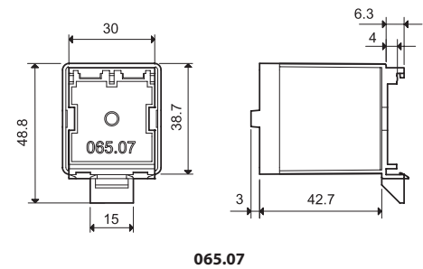
Adaptateur rail 35 mm (EN 60715) sur le dessus pour types 65.31.xxx.xxx9
