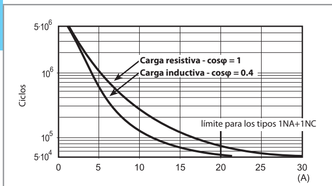
F 65 - Vida útil eléctrica (AC) en función de la carga
