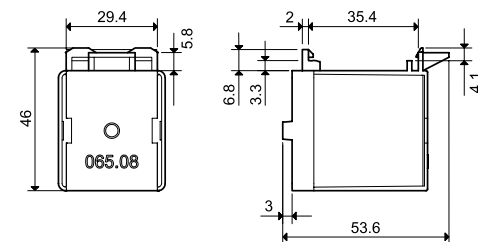
065.08
