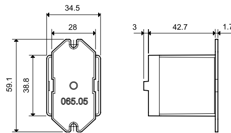
065.05
