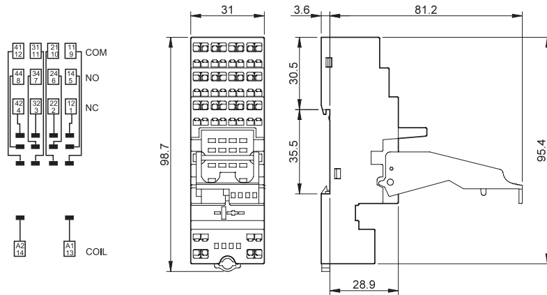
Fassung + Kammbrücke
