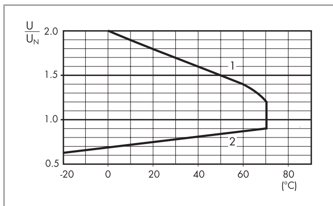
R 50 - Campo di funzionamento bobina DC in funzione della temperatura ambiente - Bobina standard (tipo 50.12)
