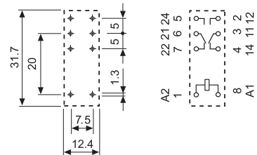
Rysunek otworów montażowych
