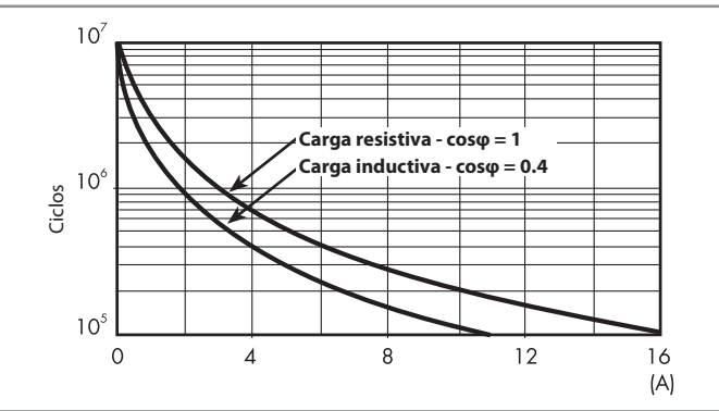
F 46 - Vida eléctrica (AC) en función de la corriente de contactos Tipo 46.61
