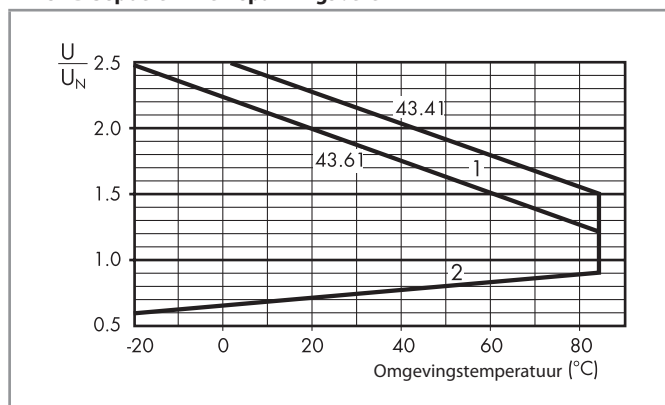
R 43 - DC spoelen -werkspanningsbereik
