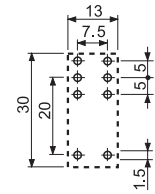
95.15.2 Вид сбоку
