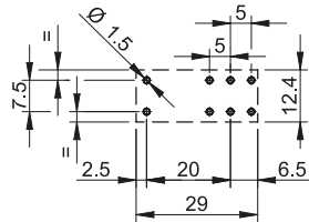
Csatlakozók nézetei
