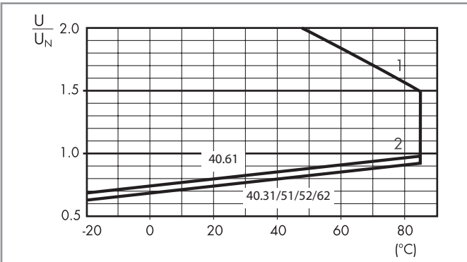
R 40 - Campo de funcionamiento de la bobina DC en función de la temperatura ambiente - Bobina sensible, tipos 40.31/51/52/61/62
