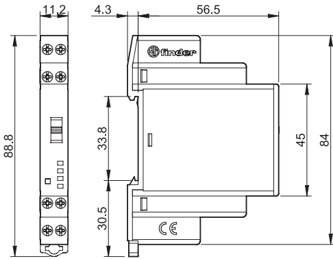
Tipo 19.91 Conexão a parafuso
