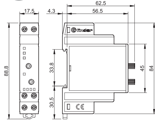
Tipo 19.3K/19.6K Conexão a parafuso Terminal KNX
