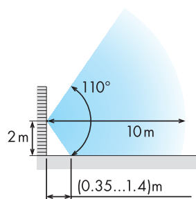
Vedere laterală
