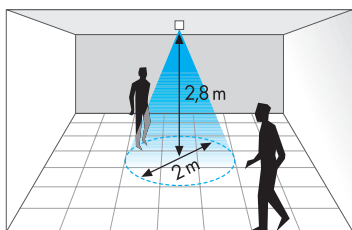
Przykład: 18.21/18.31 z ogranicznikiem zasięgu dla czujników ruchu
