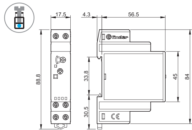
Typ 15.11 Käfigklemmen
