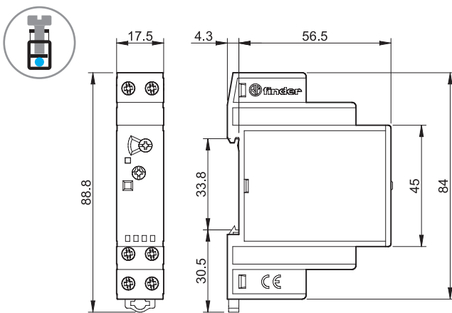
Typ 15.10 Käfigklemmen
