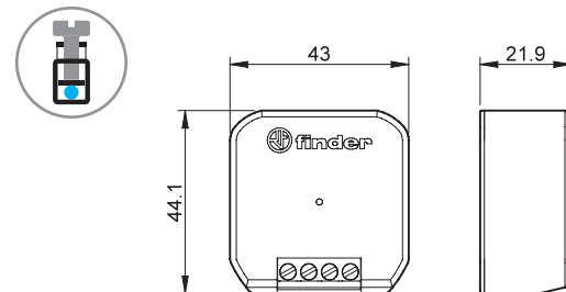
Typ 15.21 Käfigklemmen
