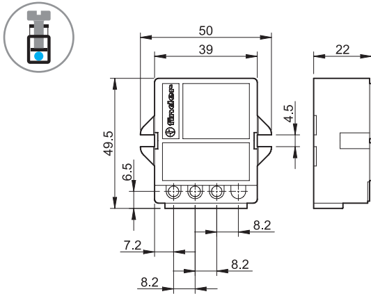
Typ 15.51 Käfigklemmen
