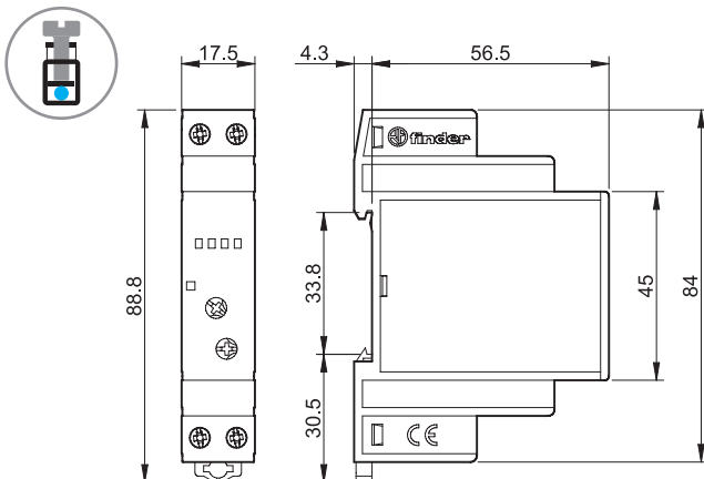
Typ 15.81 Käfigklemmen
