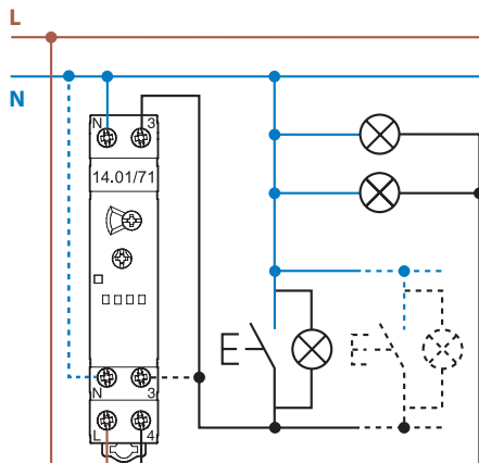
3-проводное соединение
