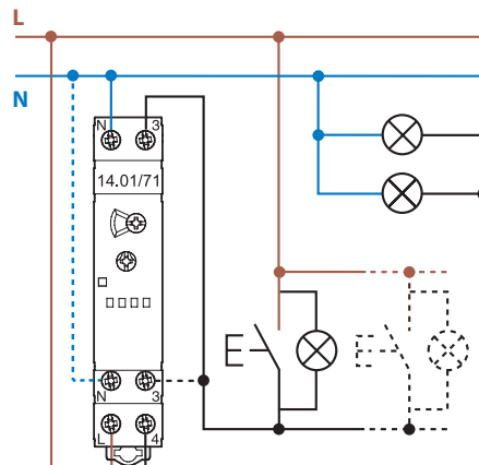
4-проводное соединение
