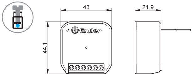
Tipo 13.21.8.230.S000 Morsetti a bussola
