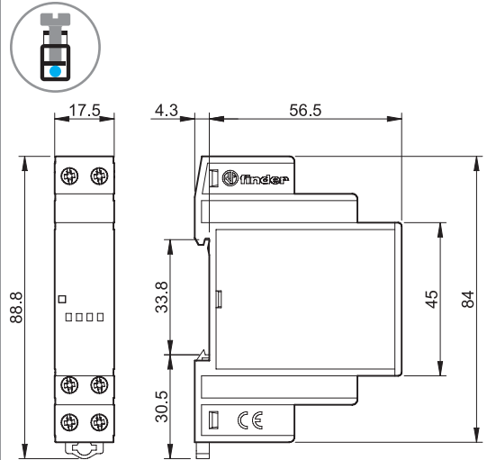
Tipo 13.81 Morsetti a bussola
