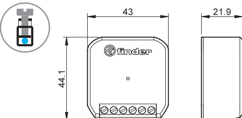
Tipo 13.21/13.22/13.52 Morsetti a bussola
