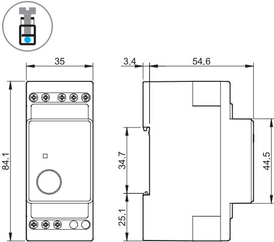
Tipo 13.11 Morsetti a bussola
