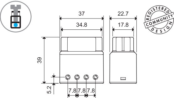
Tipo 13.21/13.22/13.52 Morsetti a bussola
