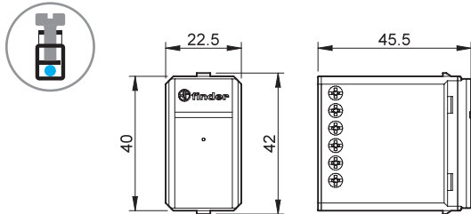
Tipo 13.72 Morsetti a bussola
