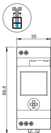
Tipurile 12.51/12.81 Terminale cu șurub
