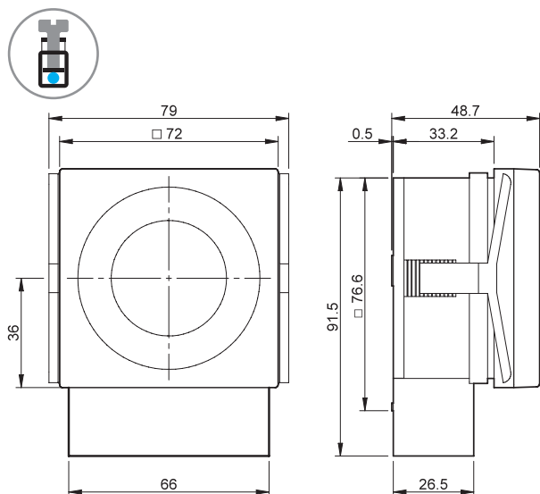
Tipul 12.31 Terminale cu șurub
