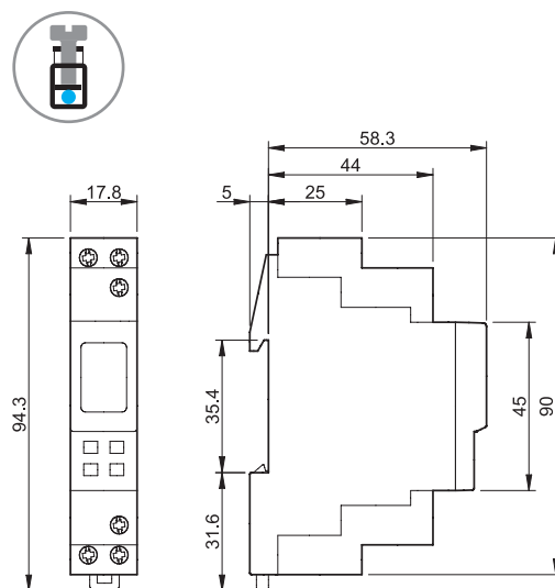
Tipul 12.71 Terminale cu șurub
