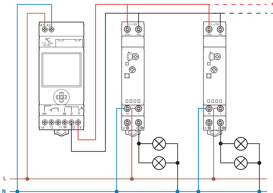
Tipul 12.A4 cu 15.11 Exemplu de aplicație cu slave dimmer Tipul 15.11 (Maxim 10)
