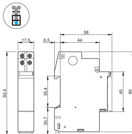
Tipul 12.11 Terminale cu șurub
