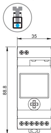
Tipul 12.B2 Terminale cu șurub
