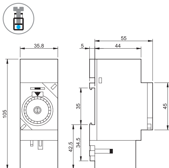
Tipul 12.01 Terminale cu șurub
