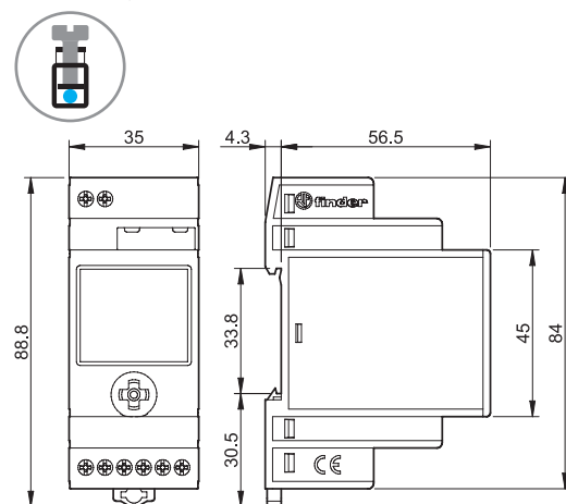
Tipurile 12.62/12.A2/12.A4 Terminale cu șurub
