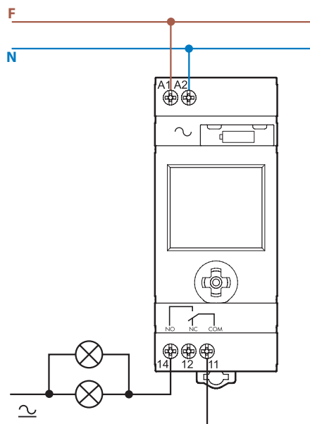
Tipo 12.51 e 12.81
