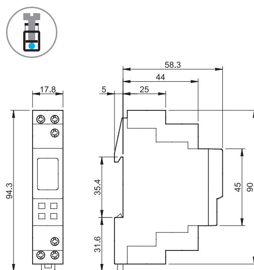
Tipo 12.71
