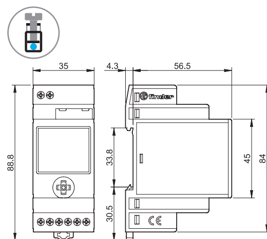
Tipi 12.62/12.A2/12.A4
