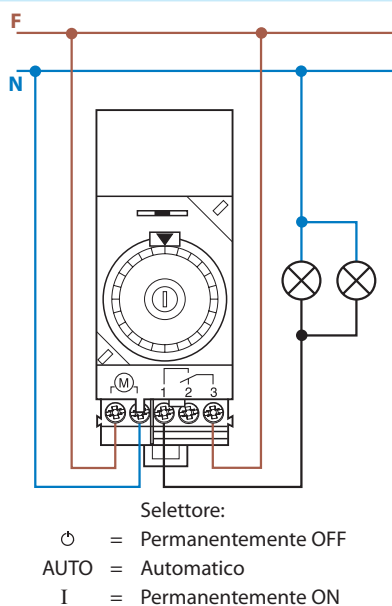
Tipo 12.01
