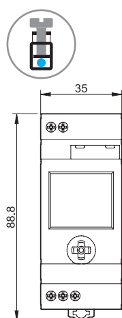
Tipi 12.51/12.81
