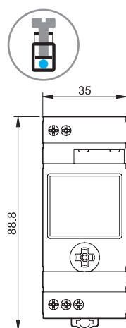
Tipi 12.61/12.A1
