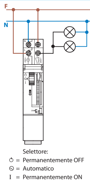
Tipo 12.11
