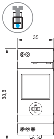
12.51/12.81 šroubové svorky
