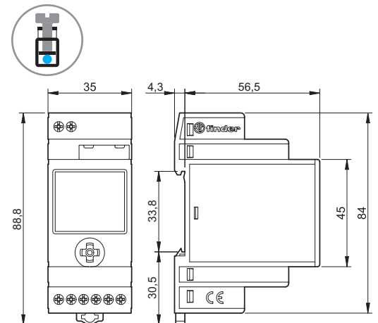
12.62/12.A2/12.A4 šroubové svorky
