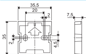
Adaptér na panel, šířka 35 mm
