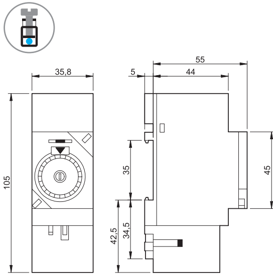
12.01 šroubové svorky
