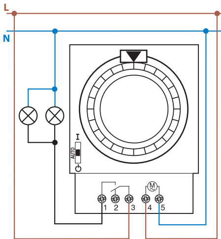
Typ 12.31
