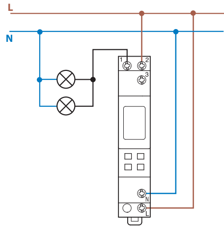
Typ 12.71
