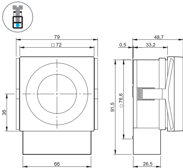
12.31 šroubové svorky
