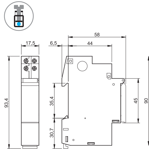
12.11 šroubové svorky
