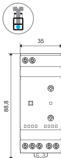
11.41 šroubové svorky
