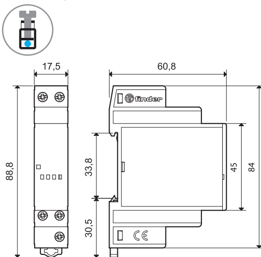
19.91 (výkonový modul pro 11.91) šroubové svorky
