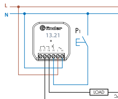
Podłączenie z przyciskiem do neutralnego
