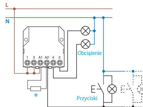
Sterowanie napięciem sieciowym współpraca z przyciskami podświetlanymi
