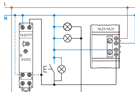
Instalacja 3-przewodowa (przyciski podłączone do neutralnego) (tylko z 18.21.8.230.0300 lub 18.31.8.230.0300)
