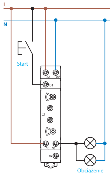
Funkcja czasowa inicjowana sygnałem start podanym na zacisk B1
