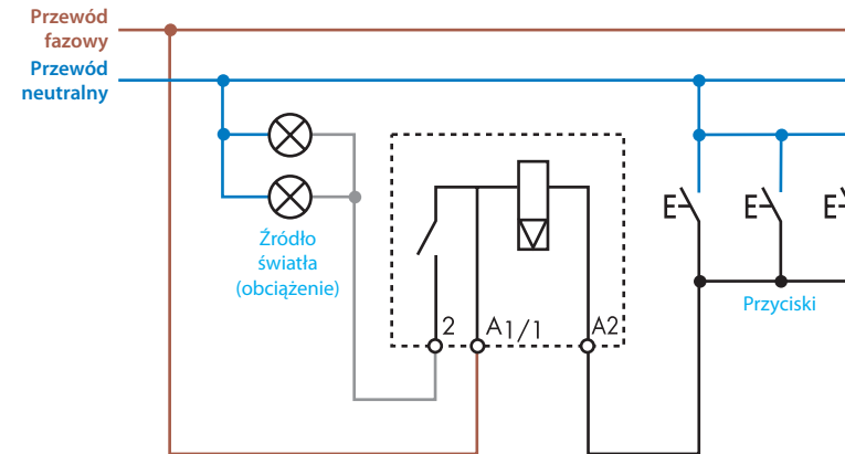
Pojedynczy obwód - System przekaźnikowy
