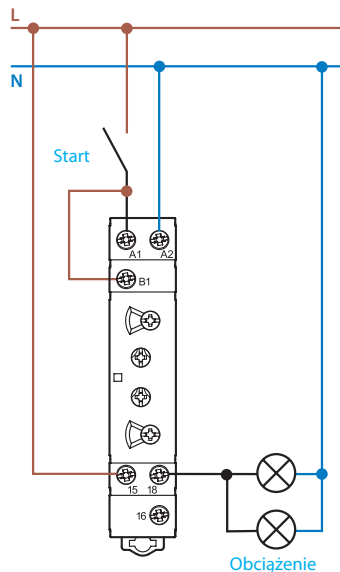
Funkcja czasowa inicjowana podaniem napięcia zasilania (A1)
