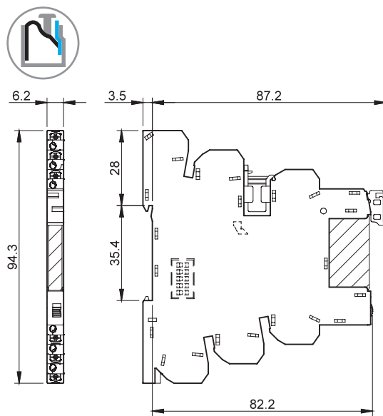
Тип 39.90 39.91 Клеммы Push-in
