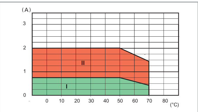
L 39-2 - AC corriente de salida en función de la temperatura ambiente 39.xx.x.xxx.8240
