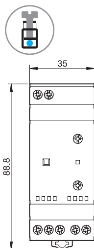
Тип 11.41 Винтовые клеммы
