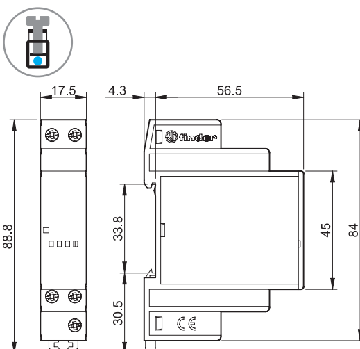
Тип 19.91 (Силовой модуль для модели 11.91) Винтовые клеммы
