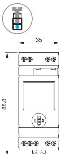
Тип 11.91 Винтовые клеммы
