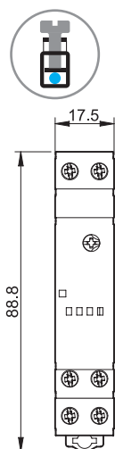
Тип 11.31 Винтовые клеммы
