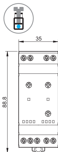
Тип 11.42 Винтовые клеммы
