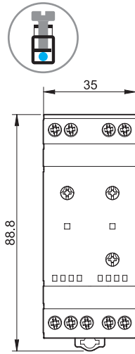
Tipo 11.42 Bornes de jaula
