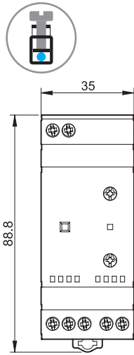
Tipo 11.41 Bornes de jaula
