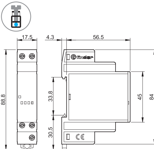
Tipo 19.91 (módulo de potencia para 11.91) Bornes de jaula
