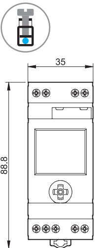
Tipo 11.91 Bornes de jaula
