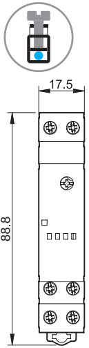
Tipo 11.31 Bornes de jaula
