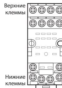
Верхние клеммы
