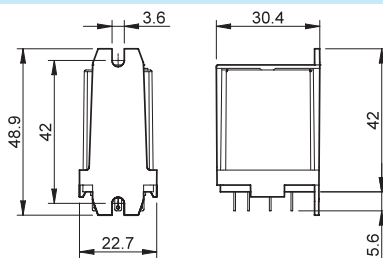
056.26 con relè
