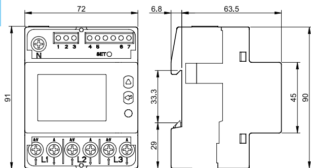
Type 7E.78.8.400.0312 Box clamp
