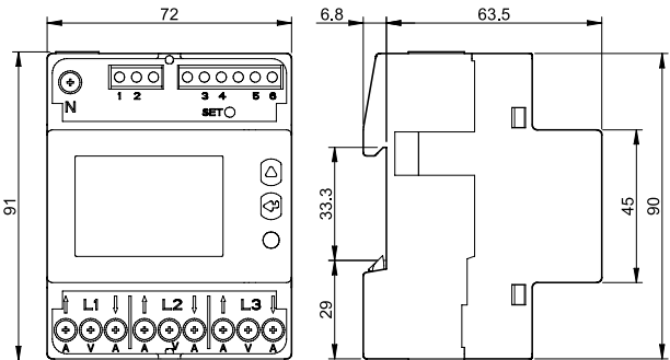
Type 7E.86.8.400.0410 Box clamp
