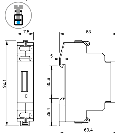
Type 7E.36.8.400.0012 Box clamp
