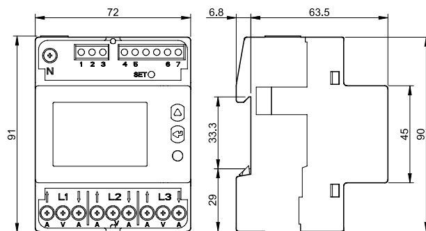
Type 7E.86.8.400.0312 Box clamp
