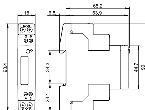
Type 7E.86.8.400.0212 Box clamp
