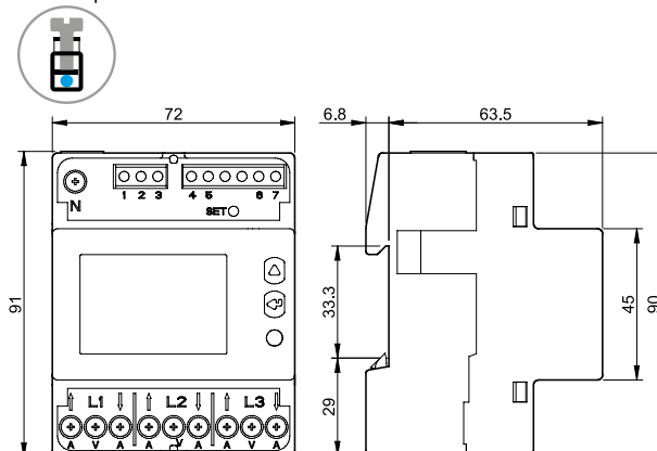
Type 7E.86.8.400.0112 Box clamp
