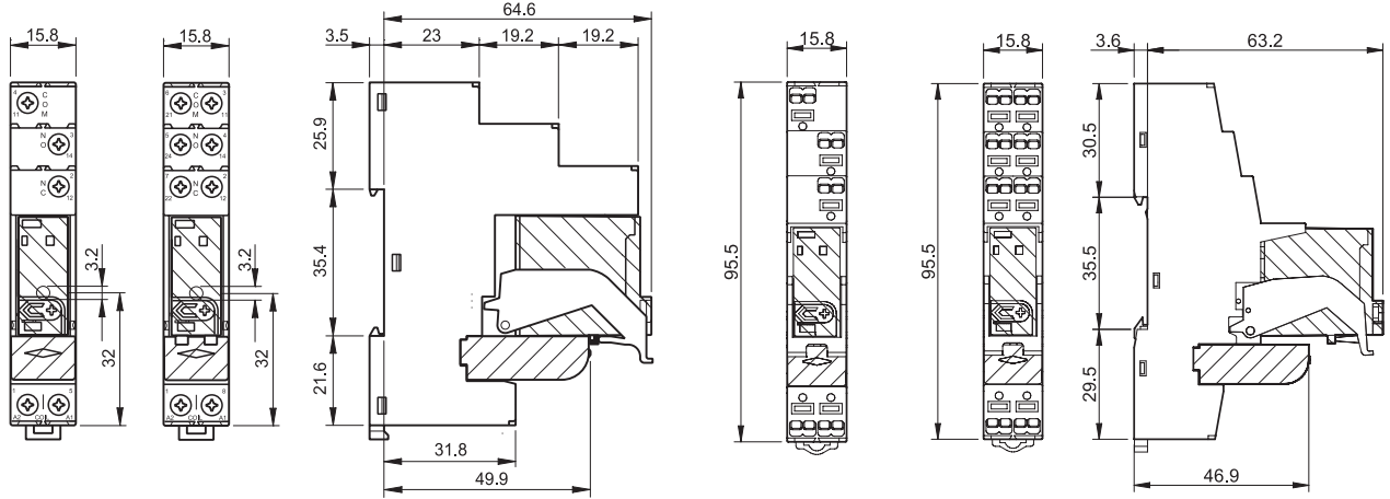
Tipo 4C.01/4C.02 Bornes de jaula
