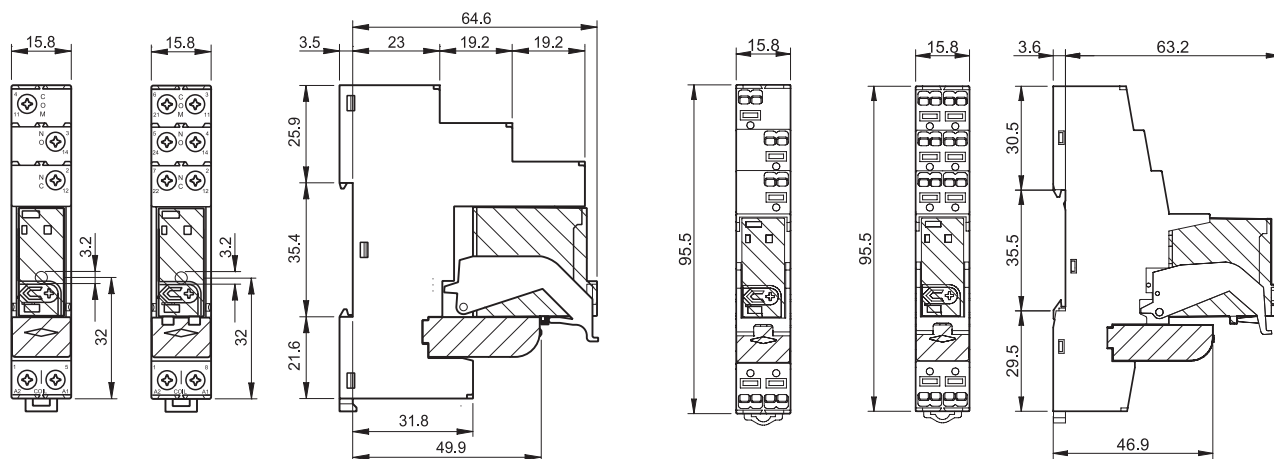
Typ 4C.01/4C.02 Käfigklemmen
