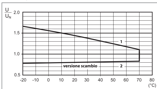
R 56 - Campo de funcionamiento de la bobina AC en función de la temperatura ambiente - 4 contactos conmutados
