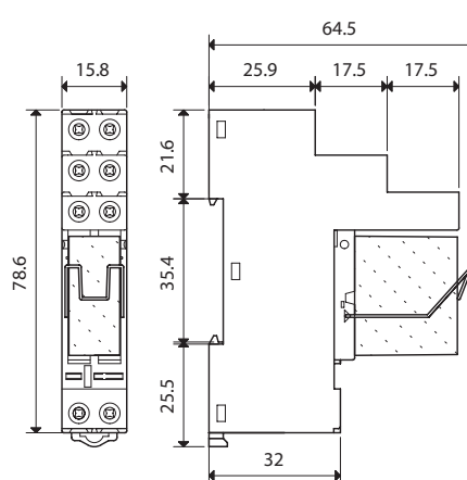
Tipo 48.12 Morsetti a bussola
