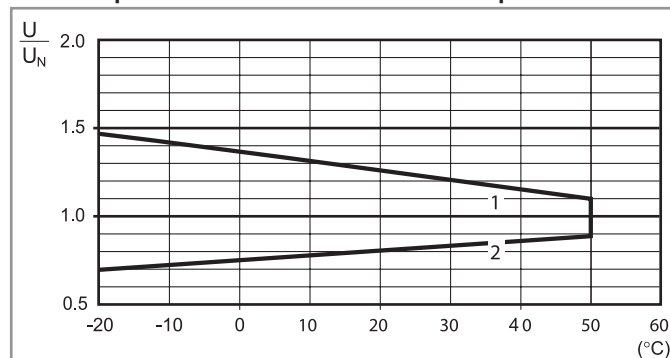
R 22 - Campo di funzionamento in funzione della temperatura ambiente
