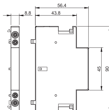
Tipo 022.63/022.65 Morsetti a vite
