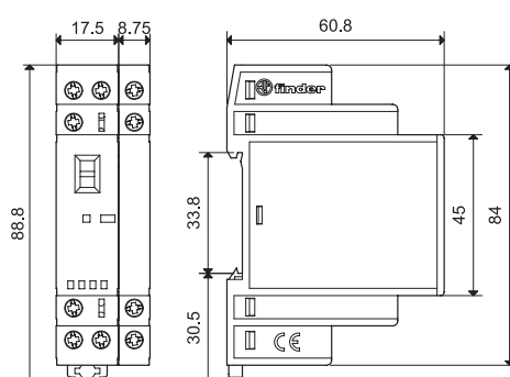
Tipo 22.W732 + 022.33/022.35 Morsetti a vite
