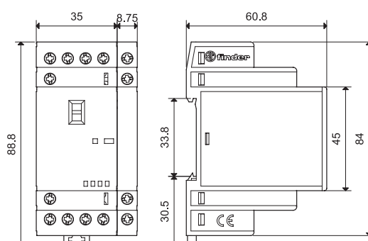
Tipo 22.34 + 022.33/022.35 Morsetti a vite
