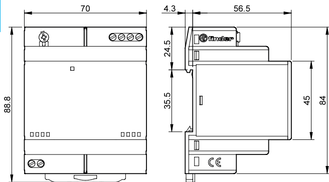
Type 78.1B Kooiklemmen
