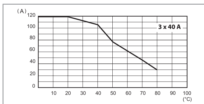
L77-23 Curentul nominal de ieșire vs. temperatura ambiantă 77.B3.x.xxx.8671
