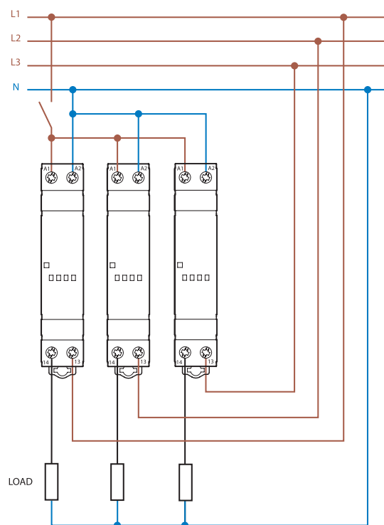
Exemplu de conexiune trifază (cu 3 x 77.01)
