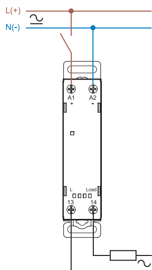
Conexiune monofazată (77.31...805x)
