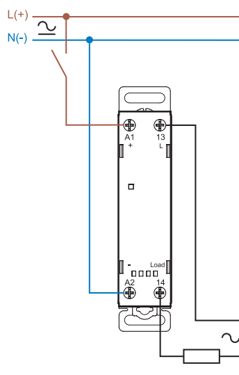
Conexiune monofazată (77.31...807x)
