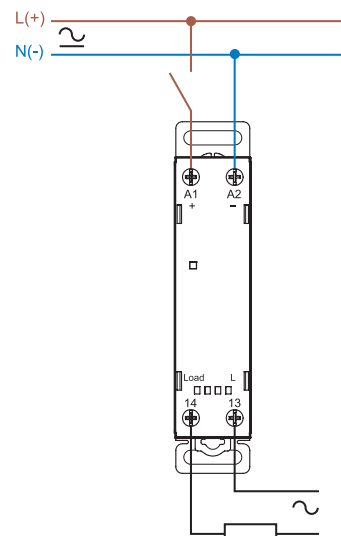
Conexiune monofazată (77.11/77.21)
